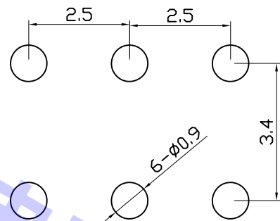
安装图 (PCB LAYOUT PLAN)
